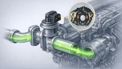
CONNETTORE PER ATTUATORE VALVOLA EGR - EXHAUST GAS RECIRCULATION (AUTOMOTIVE)
