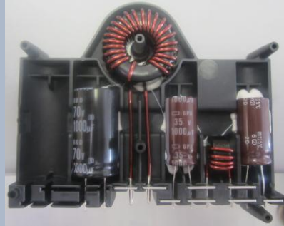
CONNETTORE FILTRO MOTORE E GAS DI SCARICO (AUTOMOTIVE)
